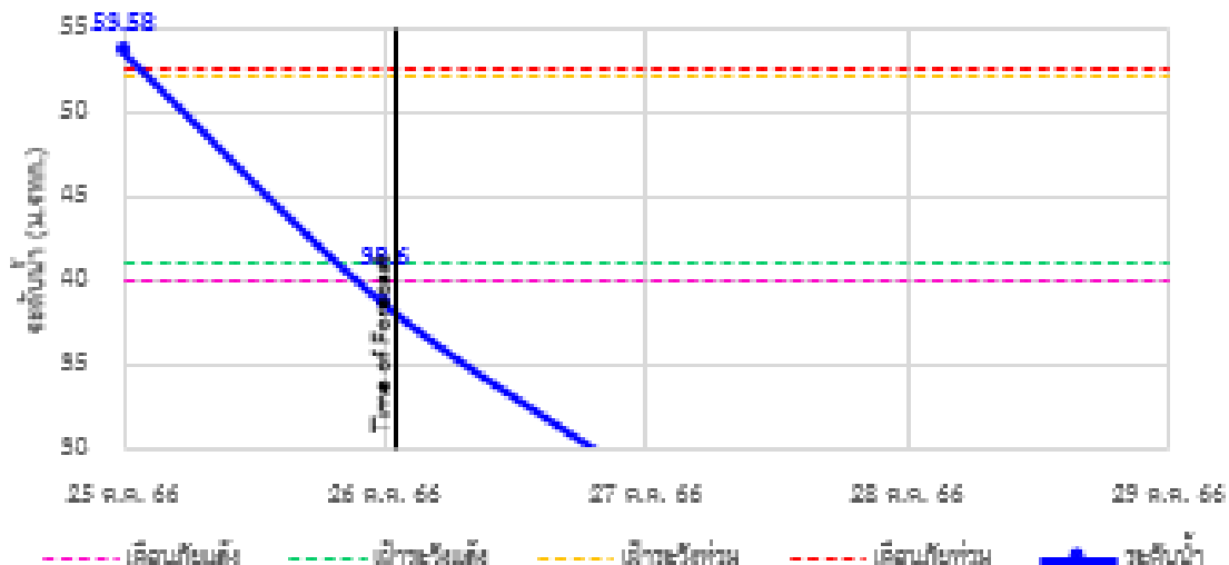
TC140605 สะพาน กาฬเจดีย์ อ.ช่องสะเคา อ.เมือง จ.กาญจนบุรี
