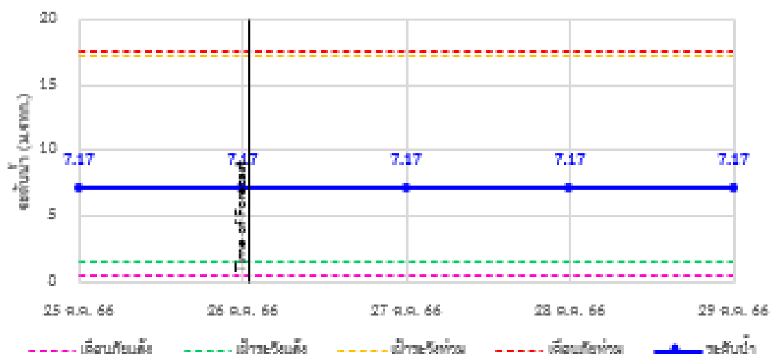
TC140102 สะพานเฉลิมพระเกียรติฯ ฝ. 60 พรรชามหาชาชีวะ จ.บ้านโป่ง จ.ราชบุรี
