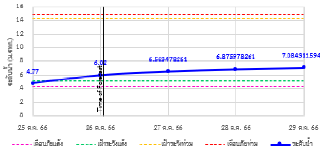
TC140101 สะพานบ้านท่าเรือ ฝ.ท่าเรือ จ.ท่ามะกา จ.กาญจนบุรี
