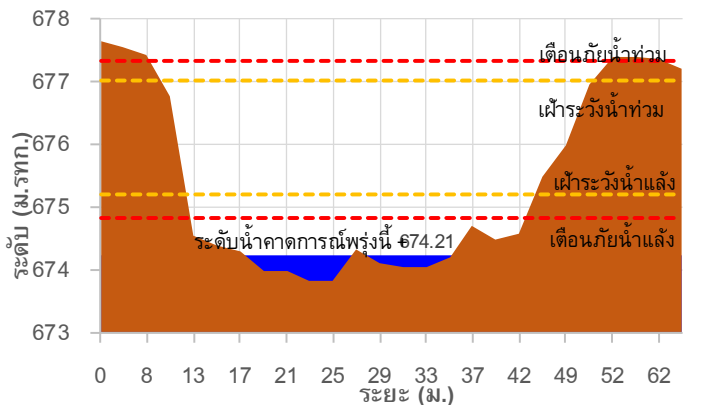
TC011202 สะพานบ้านกองก่อ
