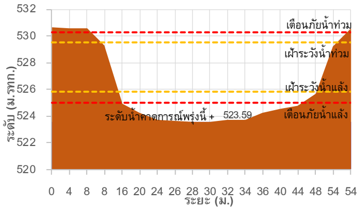
TC011008 สะพานบ้านคอนผึ้ง - บ้านห้วยสิง
